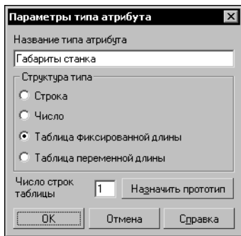
Рис. 59.2. Диалог создания типа атрибута
