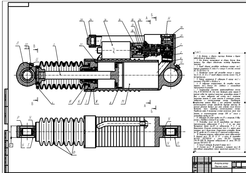
Рис. 45.1. Режим размещения технических требований
