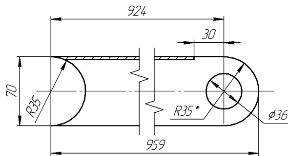
Рис. 48.4. Пример разрыва изображения
