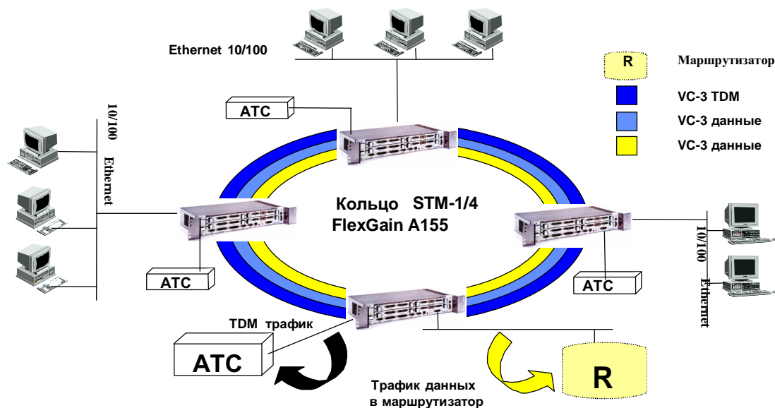
Рис. 2. Волоконно-оптическая сеть со смешанным трафиком
